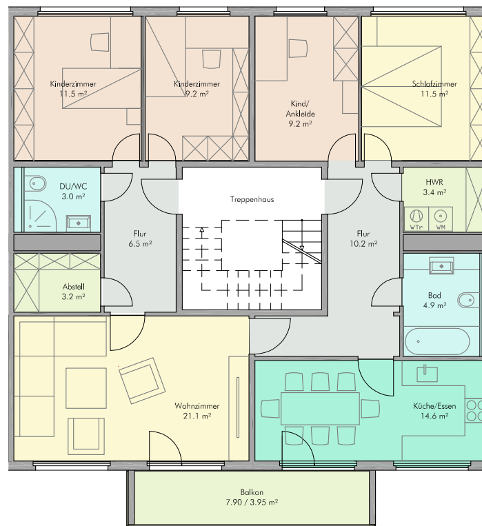
Variante 2: 3 Kinderzimmer
