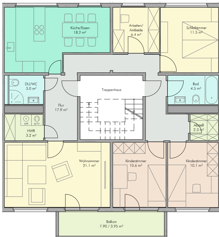
Variante 1: 2 Kinderzimmer
